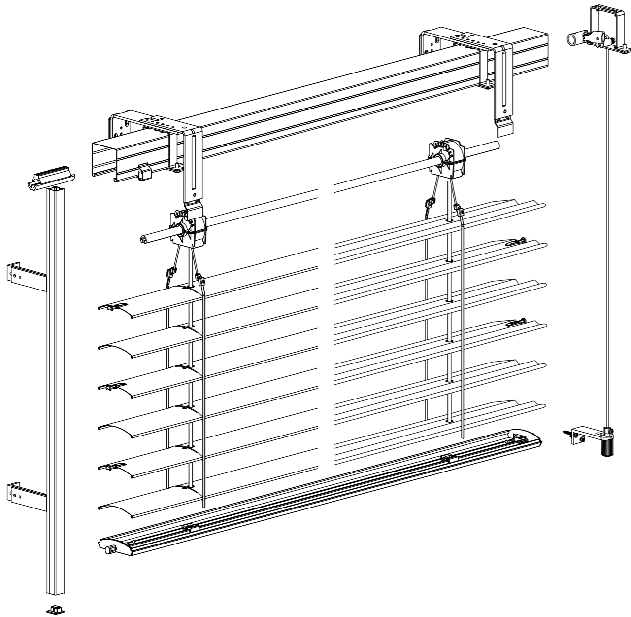
Guía Lateral 20 x 20 mm
